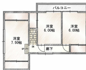
2F 平面図
